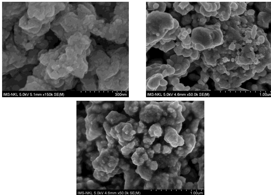
Hình 2. Ảnh SEM của mẫu LSNO (a), BTO (b) và mẫu x\text{LSNO}/(1-x)\text{BTO} với x = 0,3 (c)
