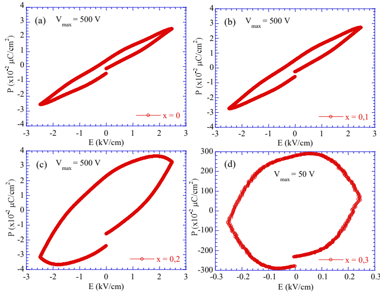
Hình 3. Đường cong điện trễ P(E) của các mẫu nanocomposite x\text{LSNO}/(1-x)\text{BTO} với x = 0 (a); 0,1 (b); 0,2 (c) và 0,3 (d). Trong đó các mẫu x = 0-0,2 được đo trong điện thế cực đại V_{\text{max}} = 500 \text{ V} và mẫu x = 0,3 đo trong điện thế cực đại V_{\text{max}} = 50 \text{ V}
