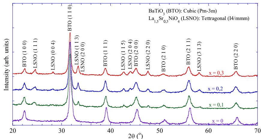
Hình 1. Giản đồ XRD mẫu bột của hệ vật liệu tổ hợp x LSNO/(1-x)BTO với x = 0; 0,1; 0,2; 0,3
