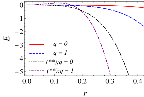
Hình 5: Sự phụ thuộc của hệ số đan rối E vào r đối với trạng thái hai mode kết hợp SU(1, 1) và trạng thái hai mode kết hợp thêm hai photon tích SU(1, 1)^{(**)} , cho h = 2 , \cos(2\varphi) = 1 và q = 0, 1 .
