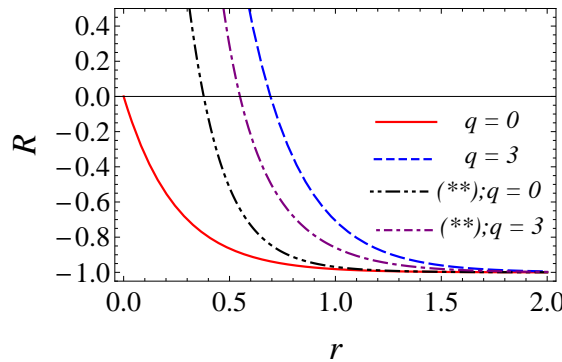
Hình 6: Sự phụ thuộc của hệ số đan rối R vào r đối với trạng thái hai mode kết hợp SU(1,1) và trạng thái hai mode kết hợp thêm hai photon tích SU(1,1)^{(**)} , cho q = 0, 3 và \cos(\varphi) = 1 .
