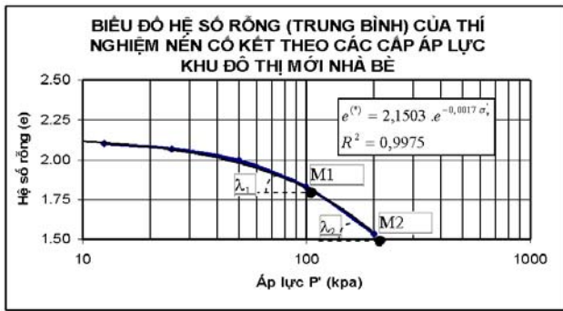
Hình 2. Đặc điểm nén ép của đất sét mềm và tương quan độ chặt theo trạng thái ứng suất.
