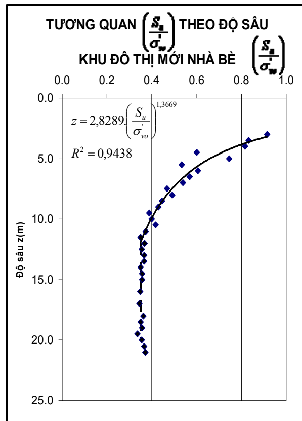
Hình 1. Biểu đồ quan hệ của ( S_u / \sigma'_{vo} ) theo độ sâu từ thí nghiệm cắt cánh
