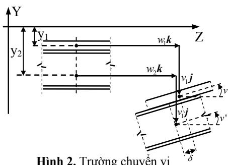
Hình 2. Trường chuyển vị
