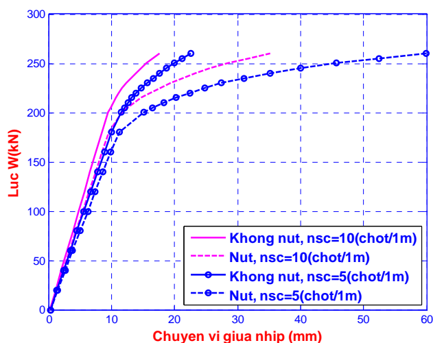
Hình 11. Chuyển vị giữa nhịp khi có xét và không xét đến bê tông bị nứt
