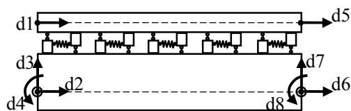
Hình 3. Phần tử dầm LH 8 bậc tự do
