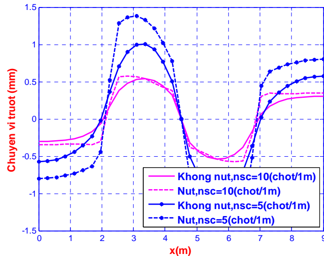
Hình 12. Chuyển vị trượt khi có xét và không xét đến bê tông bị nứt
