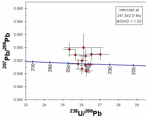
Hình 8. Biểu đồ biểu diễn giá trị tuổi đồng vị (phân tích trên khoáng vật zircon) của các đá granitoid khối Hải Vân (mẫu HVN4-Lê Đức Phúc, 2007)
