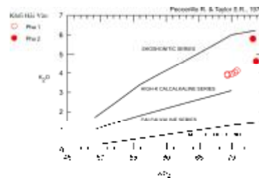
Hình 2. Biểu đồ phân chia loại magma theo Peccerillo R. & Taylor S.R., 1976
