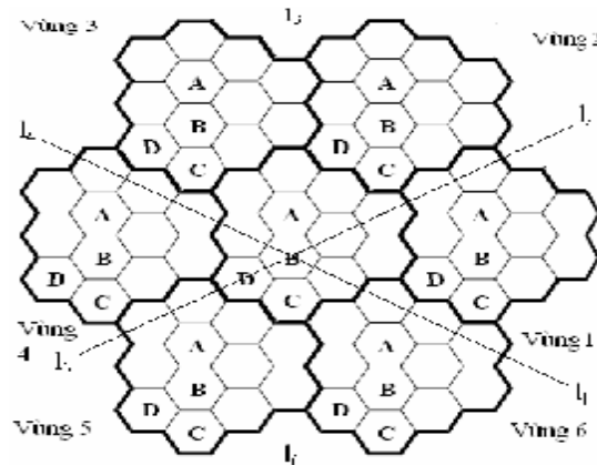
Hình 3. Nhóm Compact (i, j) = (2, 2) , N=12
