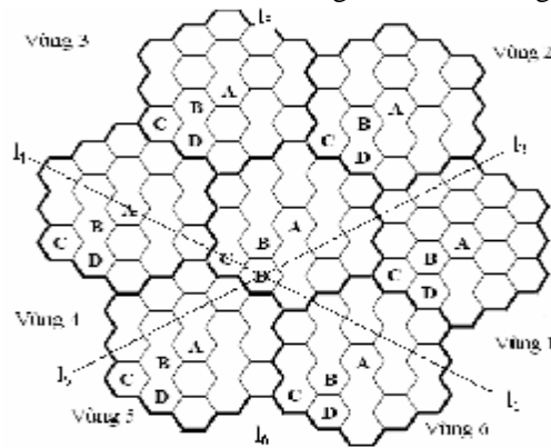
Hình 5. Nhóm Compact (i,j)=(3,2) , N=19
