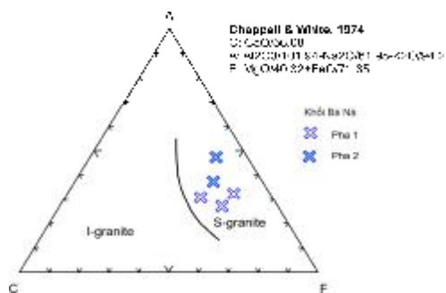
Hình 3. Biểu đồ phân chia I&S- granit
