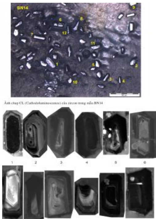
Ảnh 1. Ảnh chụp CL các hạt zircon trong mẫu BN14
