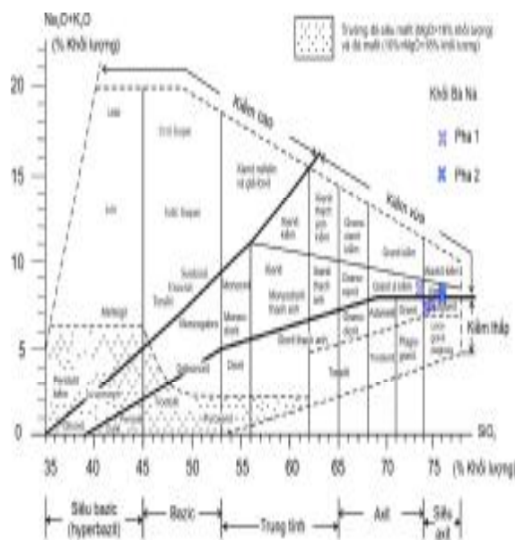
Hình 1. Biểu đồ phân loại magma theo Popov, V.S, Bogachiov O.A, 2001
