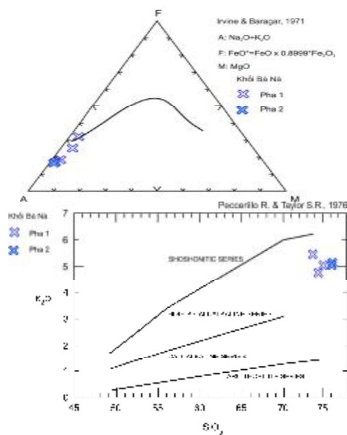
Hình 2. Biểu đồ phân chia loại magma
