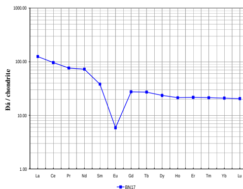
Hình 5. Biểu đồ các nguyên tố REE của granitoid khối Bà Nà được chuẩn hóa với chondrite theo Boynton, 1984
