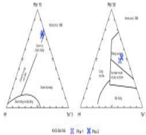
Hình 7. Biểu đồ phân chia granit theo bối cảnh kiến tạo (Harris et al., 1986)
