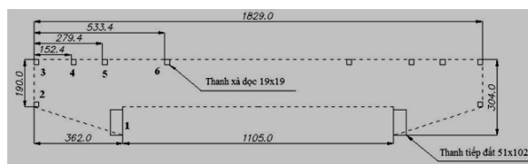
Hình 6. Mặt cắt tại sườn số 5 (giữa tàu).
