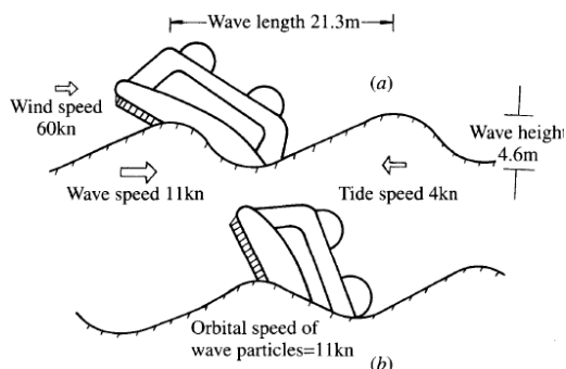
Hình 9. Hiện tượng lật do sóng ngang quá lớn.
