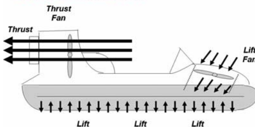
Hình 10. Bố trí hệ thống động lực đẩy và nâng.
