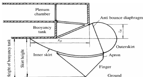
Hình 8. Thông số hình học cơ bản váy đệm khí.
