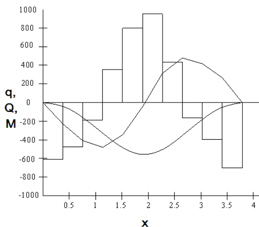
Hình 5. Lực phân bố, lực cắt và moment
