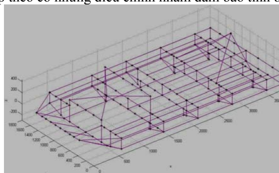
Hình 7. Mô hình tính kết cấu với phần tử dầm.
