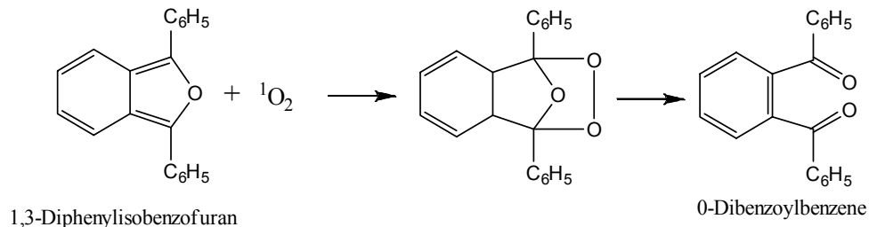
Hình 1. Phản ứng oxy hóa hợp chất 1,3-Diphenylisobenzofuran bởi 1 O 2
