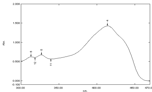
Hình 2. Phổ UV-Vis của DPBF (70 µM) trong dung môi
