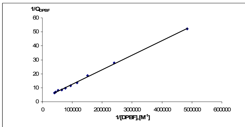
Hình 3. Đồ thị biểu diễn quan hệ giữa 1/\Phi_{DPBF} và 1/[DPBF] theo phương trình (1) của phản ứng quang oxy hóa hợp chất DPBF bằng ^1O_2 sử dụng ZnTSPc trong DMF
