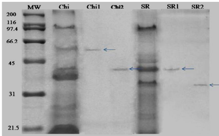
Hình 2. Kết quả SDS-PAGE hai isozyme endochitinase. Cơ chất cảm ứng là chitin huyền phù 1% (Chi1 và Chi2) và vách tế bào nấm S. rolfssii 0,5% (SR1 và SR2) cùng với mẫu thô tương ứng (Chi và SR)
