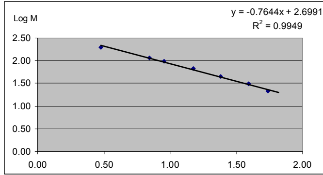
Đồ thị 3. Đường chuẩn thang protein
