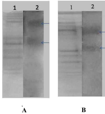
Hình 1. Các band protein trên gel polyacrylamide sau khi chạy Native-PAGE nhuộm comassive brilliant blue (lane 1) và nhuộm cơ chất đặc hiệu endochitinase trên gel agarose (lane 2) tương ứng hình A cơ chất cảm ứng là chitin huyền phù, hình B cơ chất cảm ứng là vách tế bào nấm S. rolfssii
