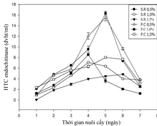
Đồ thị 2. Biến thiên HTC chitinase và endochitinase theo thời gian nuôi cấy trong môi trường TSM bổ sung các nồng độ (g/l) vách tế bào nấm S. rolfisii và P. capsici khác nhau
