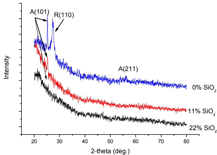
Hình 5. Phổ nhiễu xạ tia X của các màng có tỉ lệ SiO 2 khác nhau được nung ở nhiệt độ 600 0 C trong 3h.
