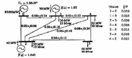
Hình 4. - Số liệu hệ thống điện 5 nút.
