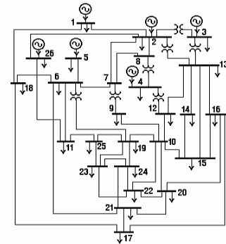
Hình 5. - Sơ đồ hệ thống điện 26 nút.
