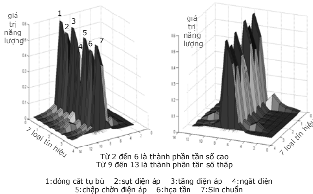
Hình 10. Biểu diễn 3D phân bố năng lượng của 7 tín hiệu
