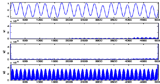
Hình 7a. Dạng sóng chập chờn điện áp và các hệ số wavelet
