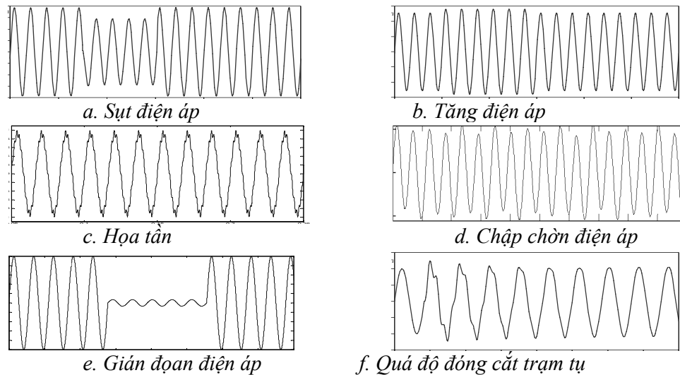
Hình 1. Dạng sóng các tín hiệu quá độ
