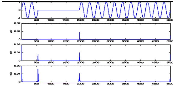
Hình 8a Dạng sóng gián đoạn điện áp và các hệ số
