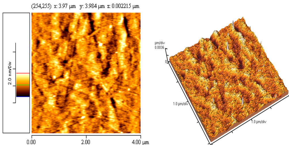
Hình 1c. TiO 2 -SiO 2 (50 % SiO 2 ) : Rms Rough: 0.4431 nm;
