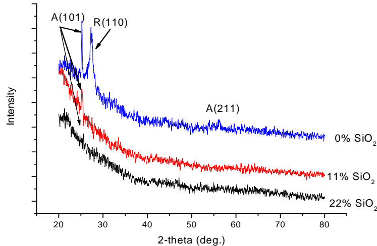
Hình 5. Phổ nhiễu xạ tia X của các màng có tỉ lệ \text{SiO}_2 khác nhau được nung ở nhiệt độ 600^\circ\text{C} trong 3h.
