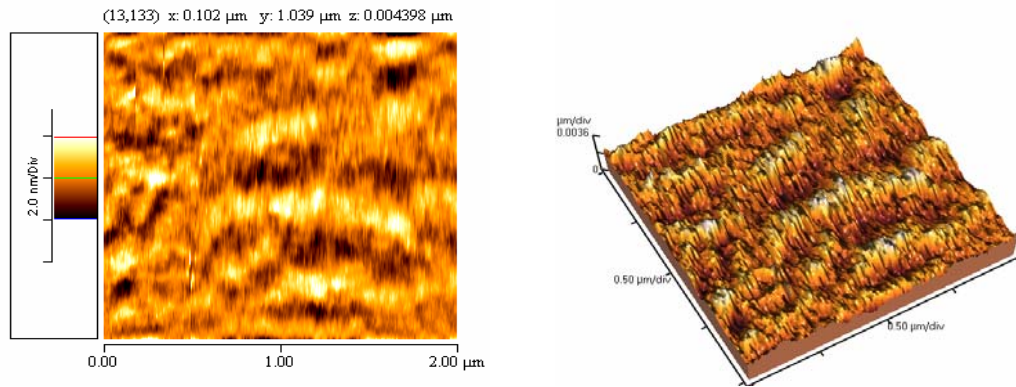
Hình 1c. TiO 2 -SiO 2 (50 % SiO 2 ) : Rms Rough: 0.4431 nm;
