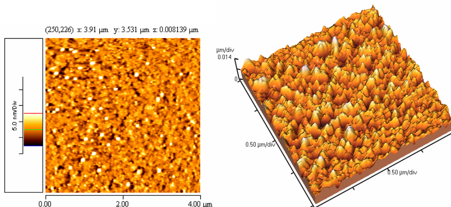
Hình 1a. \text{TiO}_2\text{-SiO}_2 (0% \text{SiO}_2 ) : Rms Rough: 6.481 (nm);
