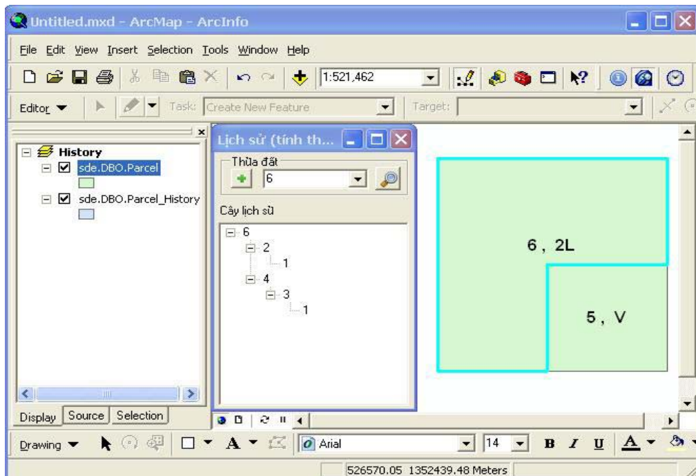
Hình 5. Kết quả truy vấn lịch sử của thửa trong ArcMap
