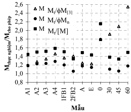
Hình 7. So sánh mômen thực nghiệm với mômen cho phép
