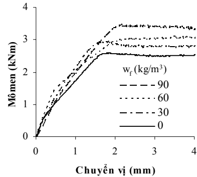
Hình 4. Quan hệ giữa mômen và chuyển vị
