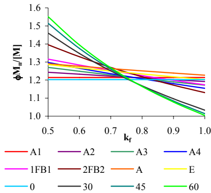
Hình 6. Quan hệ giữa \phi M_r/[M] và k_r
