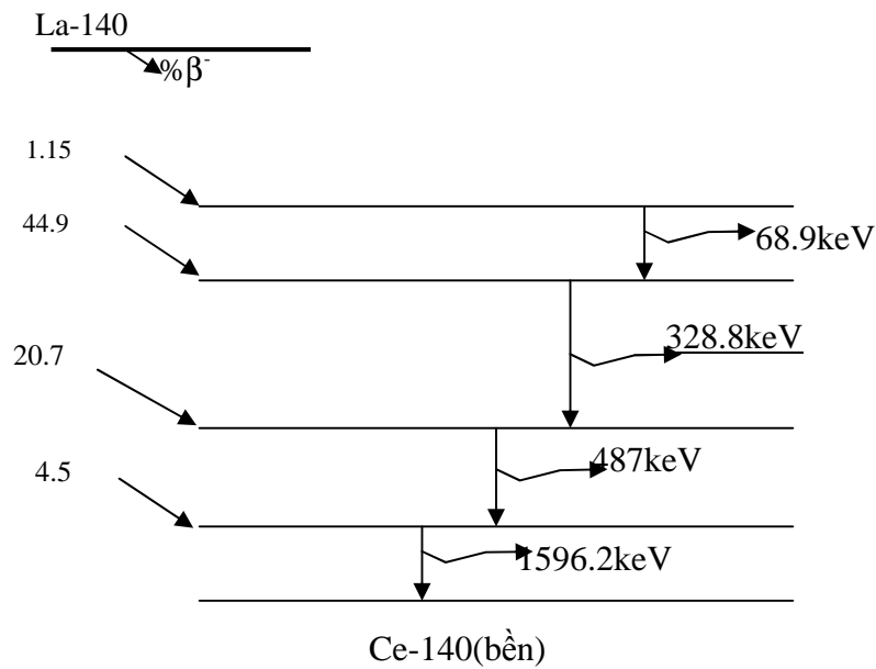
Hình 2. Sơ đồ phân rã của La-140 (chỉ lấy các mức quan tâm)
