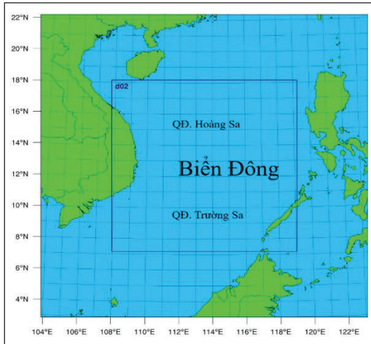
Hình 1. Miền tính sử dụng trong quá trình chạy ban đầu hóa xoáy (trái) và dự báo (phải)
