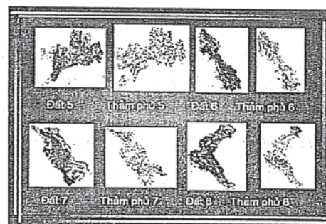
Hình 5. Bản đồ đất và thảm phủ được cắt tách của 10 tiểu lưu vực
