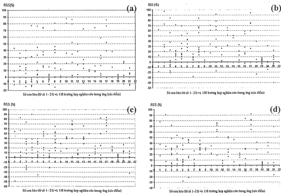
Hình 9. Phân bố chỉ số RSS cho các hạn dự báo +12 giờ (a), +24 giờ (b), +36 giờ (c) và +48 giờ (d) của 118 trường hợp nghiên cứu
