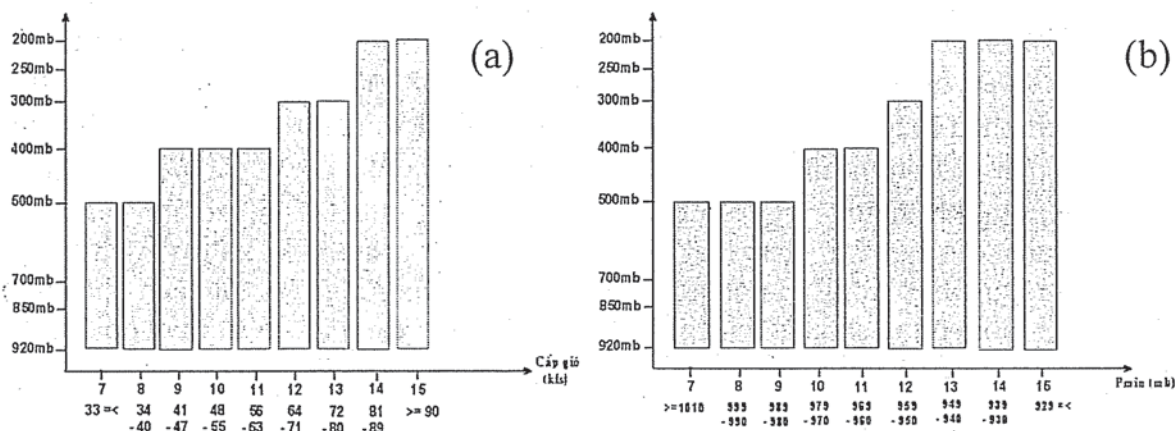
Hình 6. Mực dòng dẫn tối ưu theo cường độ bão trong phương án DLM_PP1
