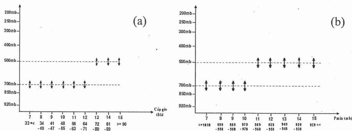
Hình 5. Mức dòng dẫn tối ưu theo cường độ bão trong phương án LEVEL ((a) phân loại theo V_{max} và (b) phân loại theo P_{min} , 1kts \approx 0,5m/s )
