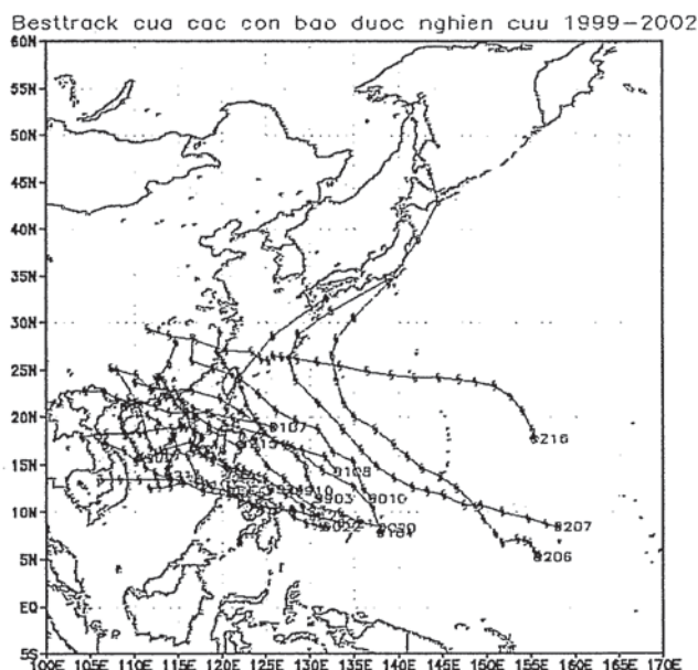
Hình 8. Quỹ đạo quan trắc của 21 cơn bão (118 trường hợp) nằm trong bộ số liệu độc lập từ năm 1999-2002
