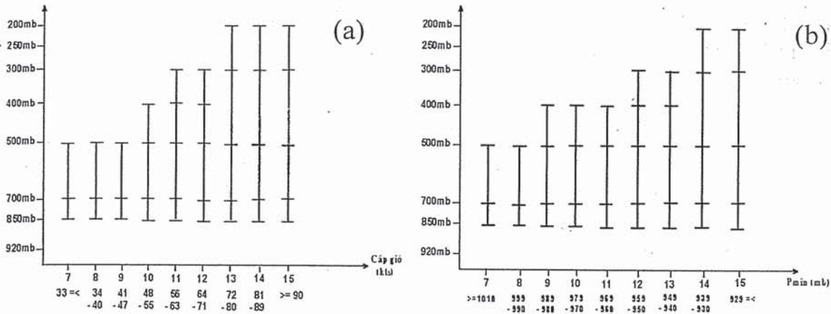
Hình 7. Mực dòng dẫn tối ưu theo cường độ bão trong phương án DLM_PP2 ((a) phân loại theo V_{max} và (b) phân loại theo P_{min} , 1kts \approx 0,5 m/s)
