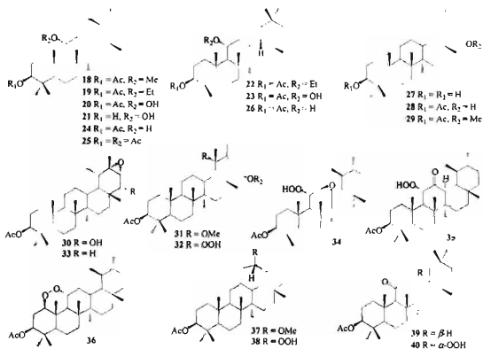
Hình 3. Cấu trúc hóa học của các hợp chất 18 - 40 (Chiang, Kuo, 2000; 2001; Kuo, Chiang, 2000).
