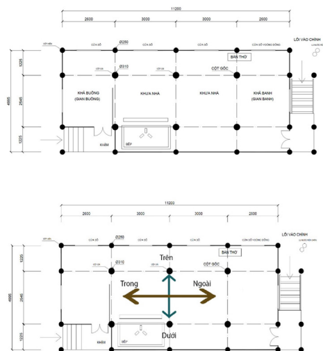
Phân chia không gian trong mặt bằng nhà ở truyền thống dân tộc Mường
