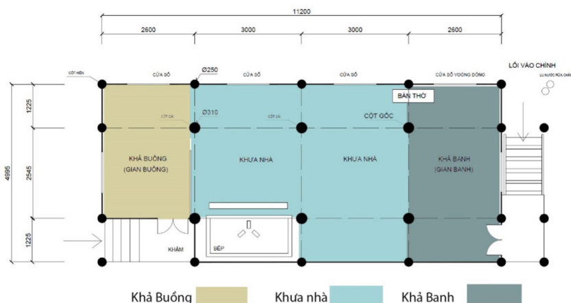
Phân chia không gian trong mặt bằng nhà ở truyền thống dân tộc Mường
