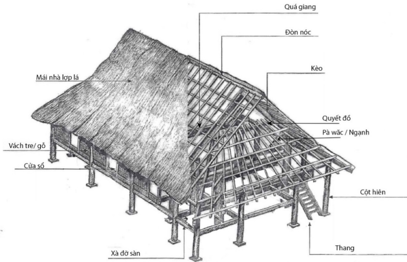
Kết cấu khung nhà ở truyền thống dân tộc Mường
