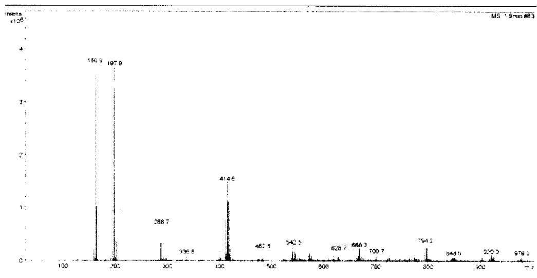
Hình 10: Các sản phẩm khử TNT bằng bột sắt (1%) ở pH = 5 với thời gian 4 giờ, sau đó hỗn hợp được oxi hóa bằng H 2 O 2 0,25% trong 4 giờ
