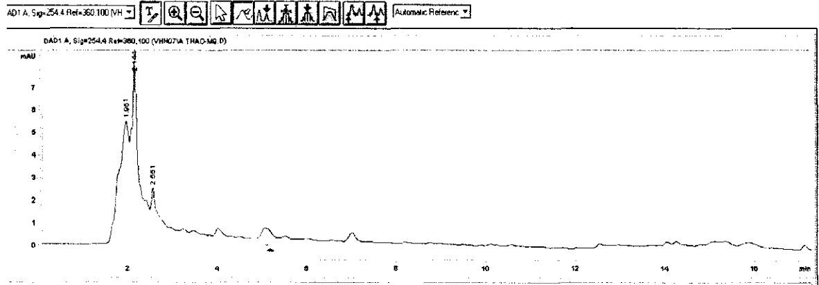
Hình 11: Phổ LC-MS của các sản phẩm khử TNT bằng Fe^0 1% (w/w, chia thành 4 liều nhỏ) ở pH = 5 với thời gian 6 giờ, sau đó hỗn hợp được oxi hóa bằng H_2O_2 0,5% (v/v) trong 8 giờ
