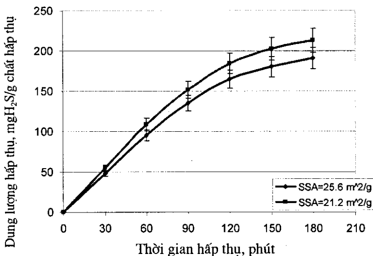
Hình 3: Tốc độ và dung lượng hấp thụ H_2S của VĐ-1 và VĐ-2 ở nhiệt độ phòng
