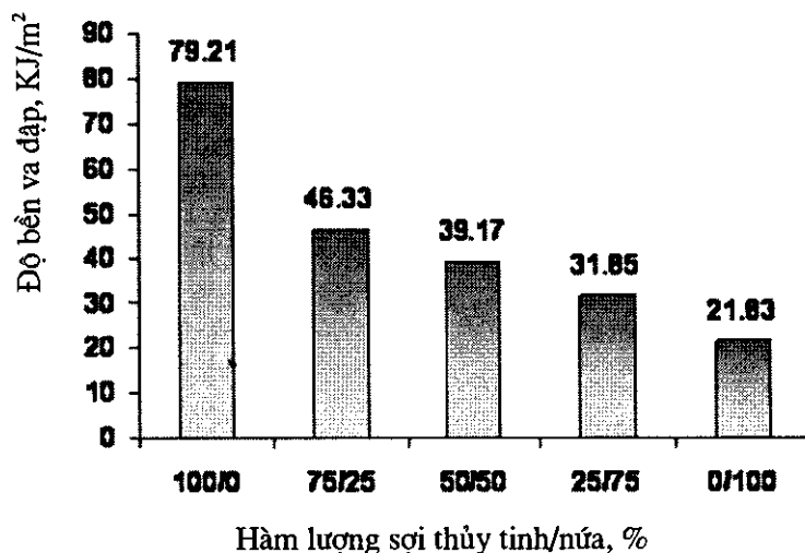
Hình 10: Ảnh hưởng của hàm lượng mat thủy tinh/nửa đến độ bền va đập của vật liệu PC
