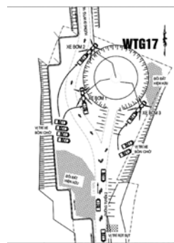
Hình 3. Mặt bằng bố trí thiết bị đổ bê tông móng
