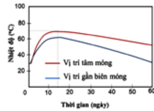
Hình 5. Minh họa kết quả đo nhiệt độ trong khối móng
