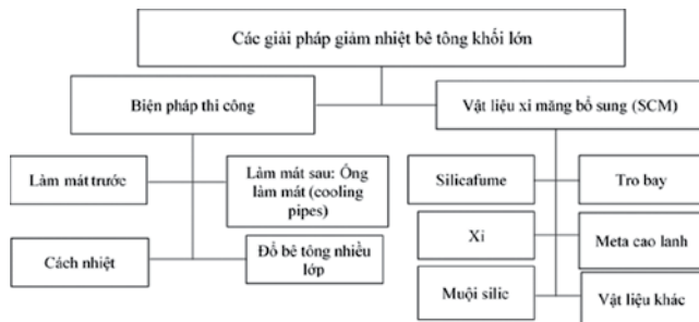
Hình 1. Các giải pháp giảm nhiệt cho bê tông khối lớn [2]
