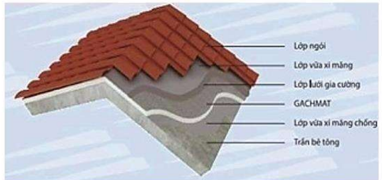
Hình 9 Gạch AAC cách âm, cách nhiệt, trích đoạn cấu tạo mái ngói dán sàn bê-tông cách nhiệt (gạch mát xốp PU)
