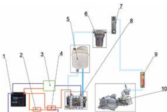
Hình 3.2. Sơ đồ cấp khí HHO
