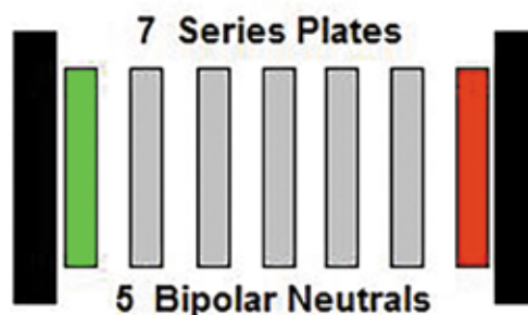
Hình 3.1. Sơ đồ bố trí bản cực
