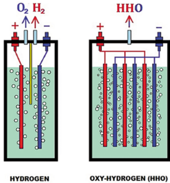
Hình 1.2. Sơ đồ nguyên lý điện phân tạo hydrogen và điện phân tạo khí HHO
