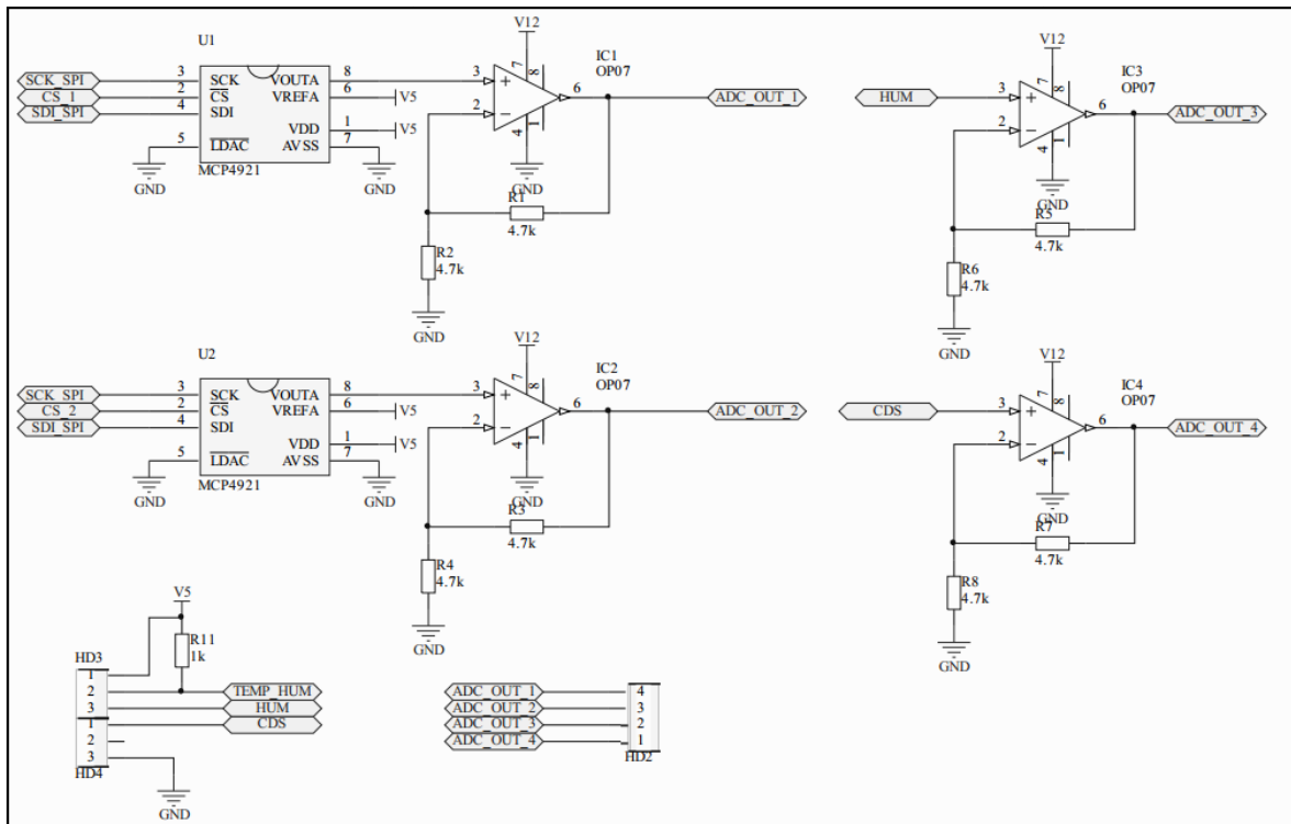
Hình 7b. Mạch khuếch đại thuật toán
