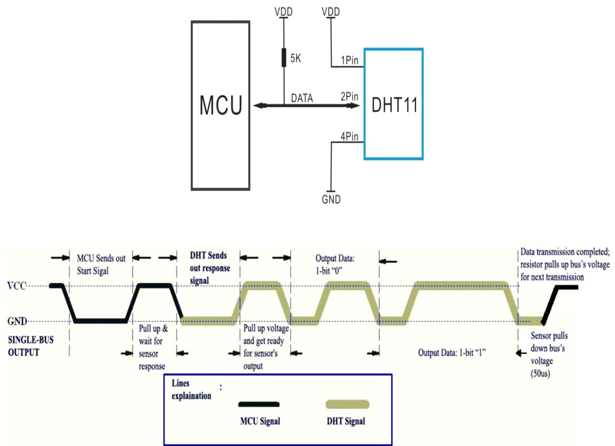
Hình 2. Ứng dụng với MCU (Micro-computer Unite) đọc dữ liệu
