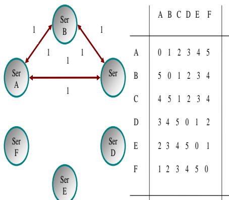
(a) K=6 ; V=6 ; \text{DCSS} = 0.2
