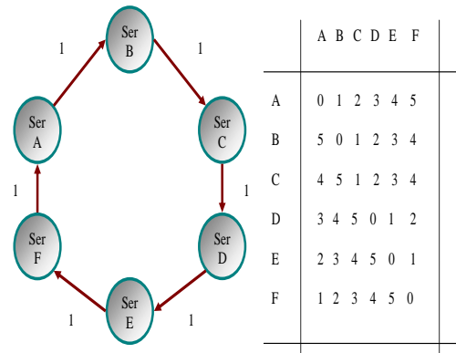
(b) K=6 ; V=6 ; \text{DCSS} = 0.6
