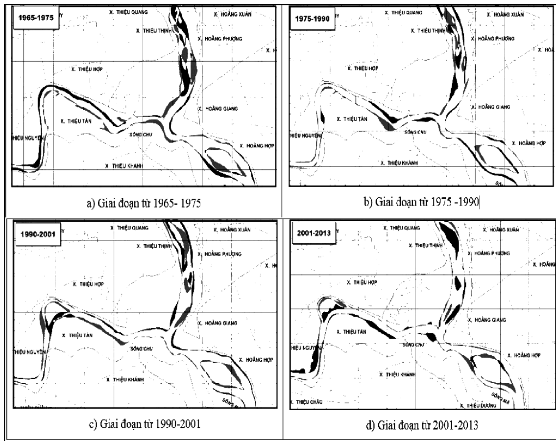
Hình 1. Tổng hợp diễn biến khu vực hợp lưu Giàng từ năm 1965- 2013
