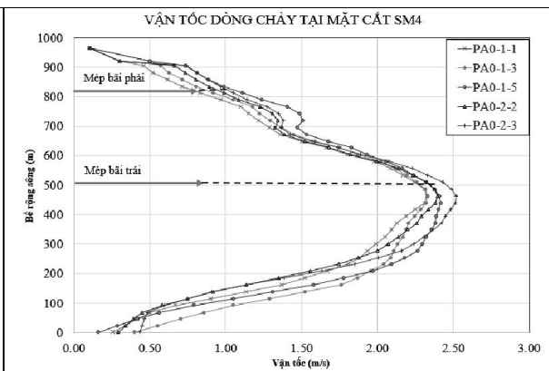
Hình 6. Vận tốc dòng chảy tại mặt cắt 4 SM4 theo các kịch bản
