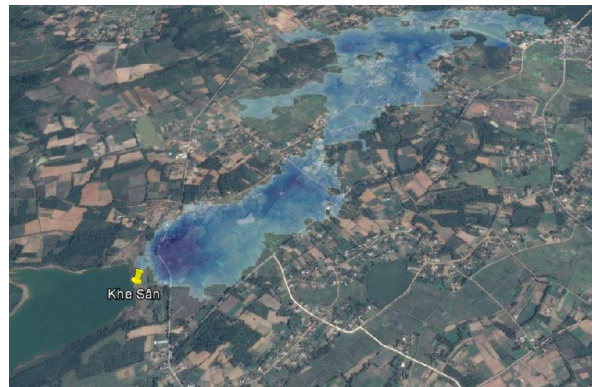
Hình 6. Khu vực ngập lụt hạ du hồ chứa
