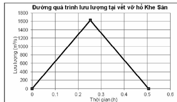
Hình 3. Đường quá trình lưu lượng tại vết vỡ hồ Khe Sân
