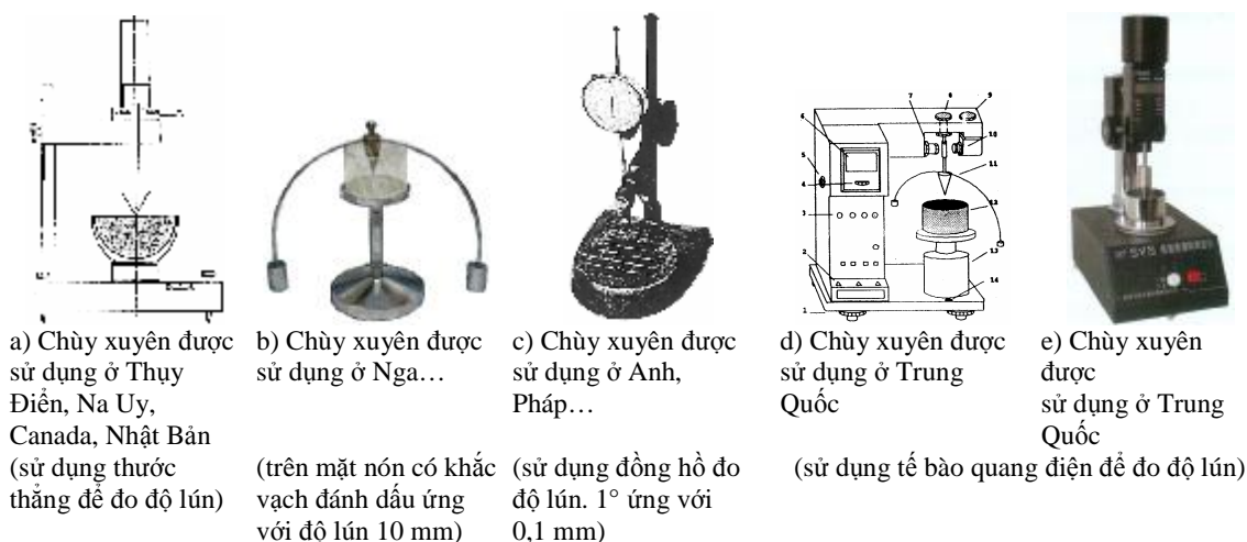
Hình 2: Khuyh hướng phát triển các loại chùy xuyên đang được sử dụng ở các nước
