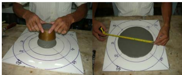
Hình 3. Thí nghiệm chảy xoè Haegermann dùng xác định tính tự đầm của hỗn hợp bê tông nền
