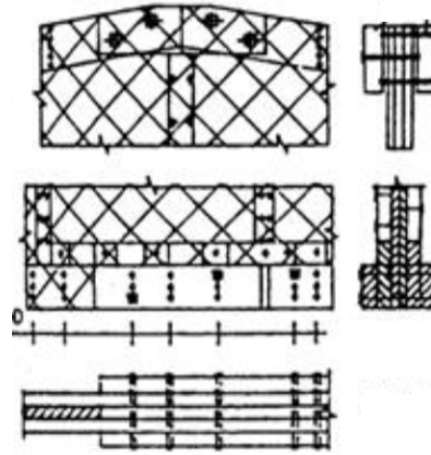
Hình 5. Chi tiết dầm ván ghép
