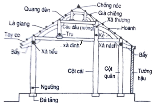
Hình 1. Khung gỗ nhà dân gian
