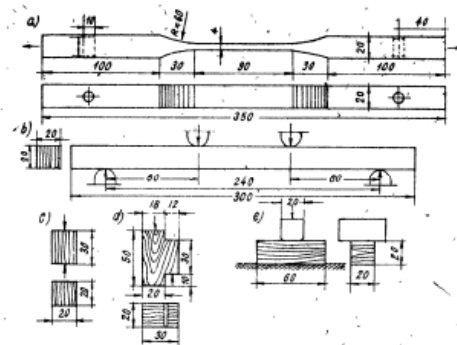
Hình 2. Các loại mẫu thử nghiệm
