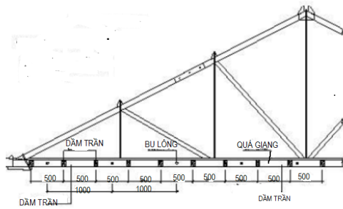
Hình 4. Giàn vì kèo có thanh đứng bằng thép
