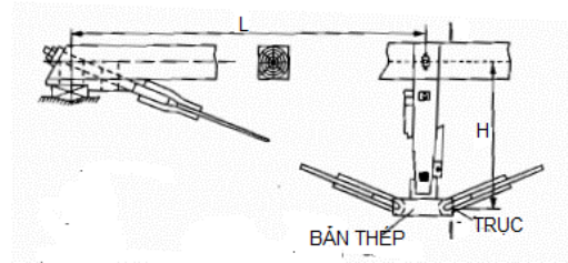
Hình 6. Chi tiết kim loại trong giàn thép-gỗ
