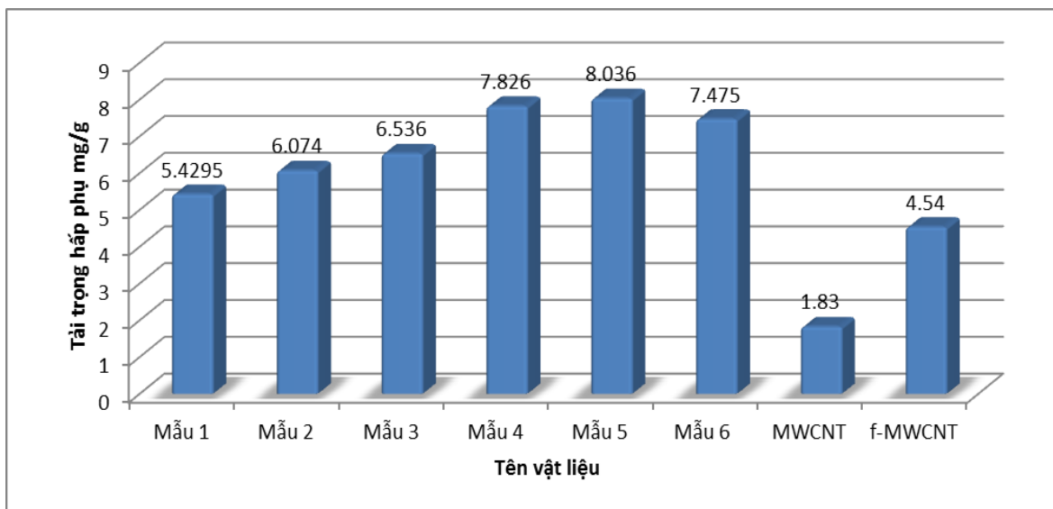
Hình 1: Tải trọng hấp phụ arsen của các vật liệu
