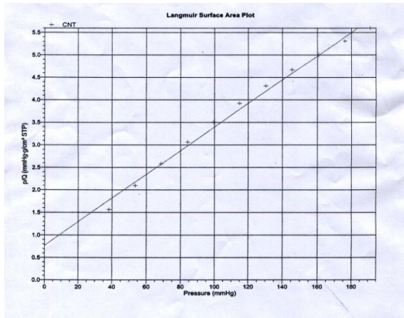
Hình 4: Đồ thị BET của MWCNs
