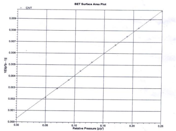
Hình 5: Đồ thị BET của f-MWCNTs
