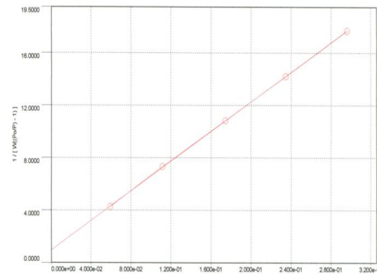
Hình 7: Đồ thị BET của m-ZrO 2 -f-MWCNTs
