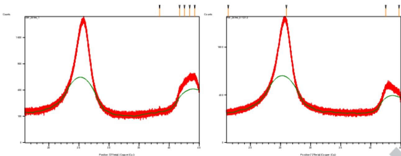
Hình 2. Kết quả đo XRD của a. MWCNTs; b. f-MWCNTs
