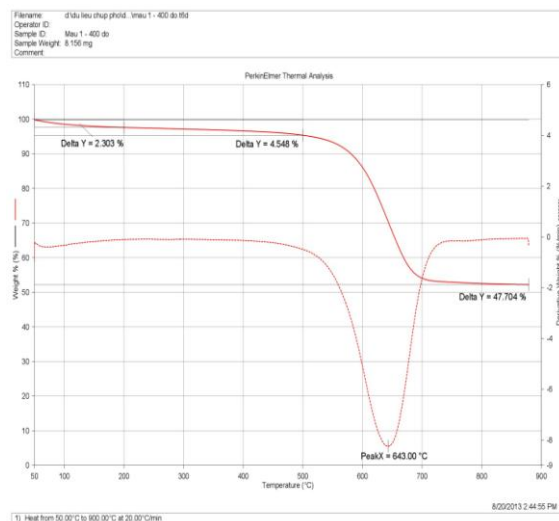
Hình 10. Kết quả TGA của mẫu M5 ở 400^\circ\text{C}
