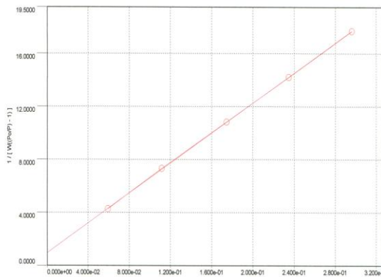
Hình 6: Đồ thị BET của t-ZrO 2 -f-MWCNTs
