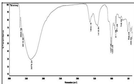
Hình 1. Phổ FTIR của lớp đất sét ủ trướng bắc thảo
