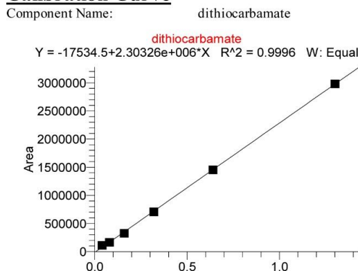
Hình 5. Đường chuẩn CS 2 trong isooctane
