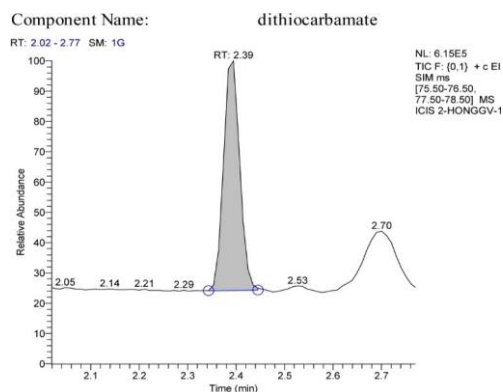
Hình 4. Sắc ký đồ GC của CS 2
