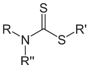
Hình 3. Cấu trúc dithiocarbamate
