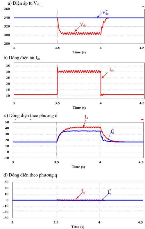
Hình 5. Kết quả mô phỏng dùng bộ điều khiển PI trong trường hợp tăng tải và giảm tải. (a) Điện áp tụ DC. (b) Dòng điện tải. (c) Dòng điện theo phương d. (d) Dòng điện theo phương q.
