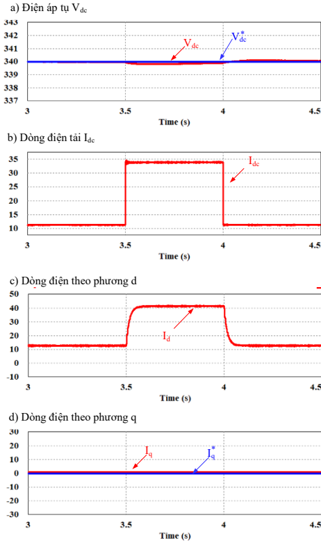
Hình 4. Kết quả mô phỏng dùng bộ điều khiển đề xuất trong trường hợp tăng tải và giảm tải. (a) Điện áp tụ DC. (b) Dòng điện tải. (c) Dòng điện theo phương d. (d) Dòng điện theo phương q.
