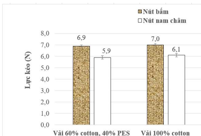
Hình 5. Biểu đồ so sánh lực kéo trong thí nghiệm đo độ bám dính
