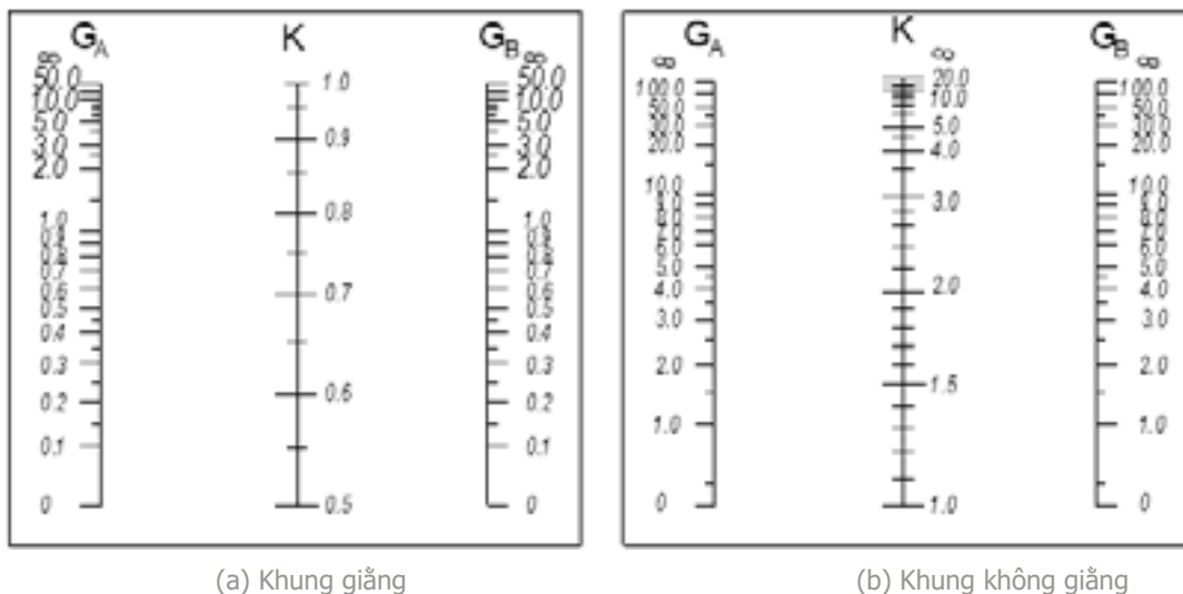
Hình 3. Biểu đồ xác định chiều dài tính toán của cột trong khung
