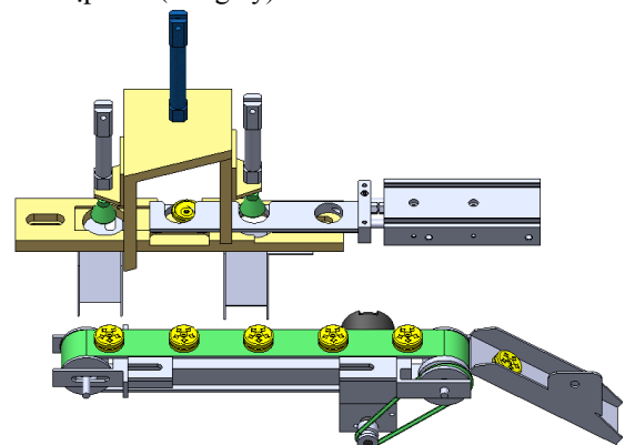
Hình 10. Cụm cơ cấu băng tải đưa kẹo
