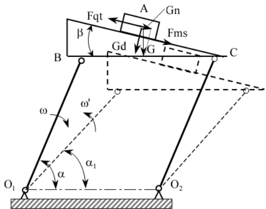
Hình 4. Sơ đồ phân tích lực dịch phôi theo quán tính trên mặt phẳng nghiêng [4]
