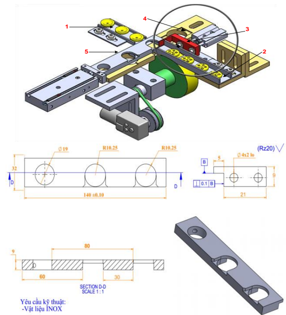
Hình 8. Cơ cấu khuôn định vị
