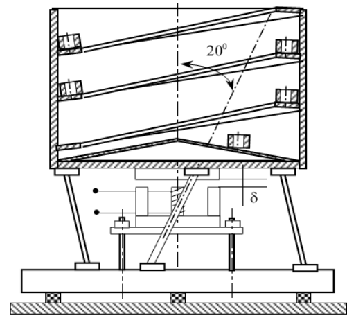
Hình 5. Phễu cấp phôi kiểu rung động
