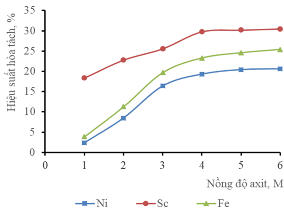
Hình 1. Ảnh hưởng của nồng độ axit đến hiệu suất thu hồi Ni, Sc và Fe
