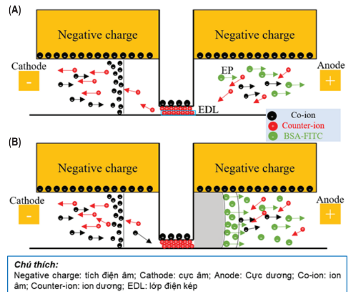
Hình 2. Nguyên lý của hiệu ứng phân cực nồng độ ion (ICP) thông qua màng chọn lọc ion: (A) Sự hình thành lớp điện kép (EDL) tại thành của kênh nano; (B) Sự tích tụ protein bị ảnh hưởng bởi dòng điện thẩm (EOF).
