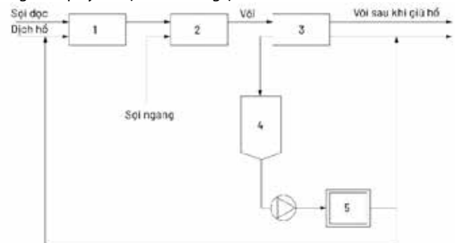
Hình 3. Nguyên lý phương pháp siêu lọc thu hồi
