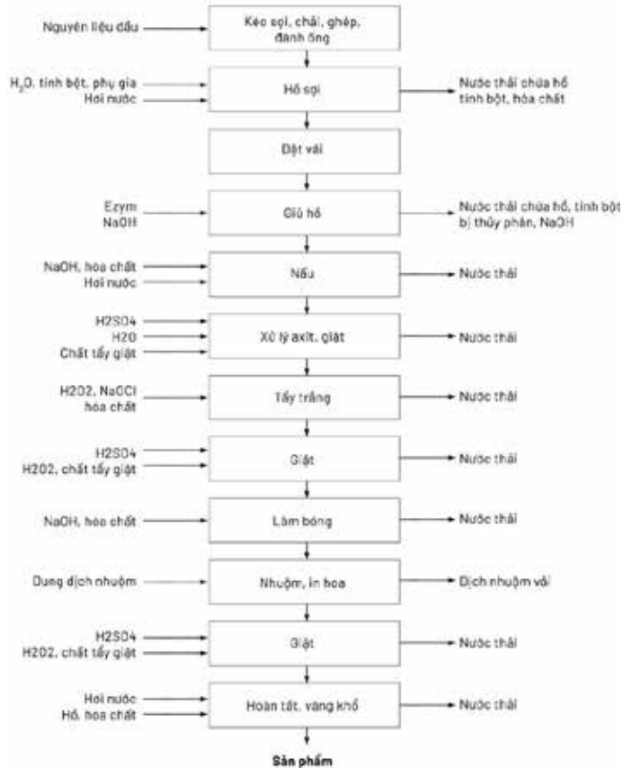
Hình 1. Sơ đồ nguyên lý công nghệ dệt nhuộm và các nguồn nước thải [1]
