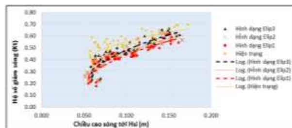
Hình 8: Biến thiên K_t khi thay đổi hình dạng cấu kiện Reffball từ Elip 1 đến Elip 3
