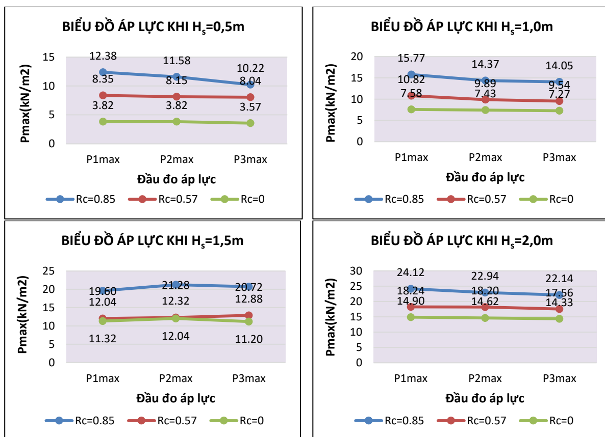
Hình 15: Biểu đồ áp lực tương ứng với các tổ hợp thí nghiệm khác nhau
