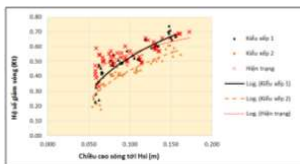
Hình 6: Biến thiên hệ số giảm sóng khi thay đổi kiểu xếp khác nhau
