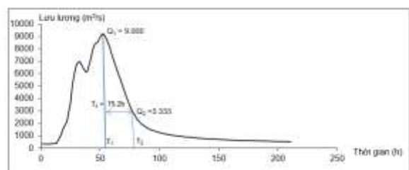
Hình 2: Biểu đồ đường quá trình lưu lượng lũ đến
