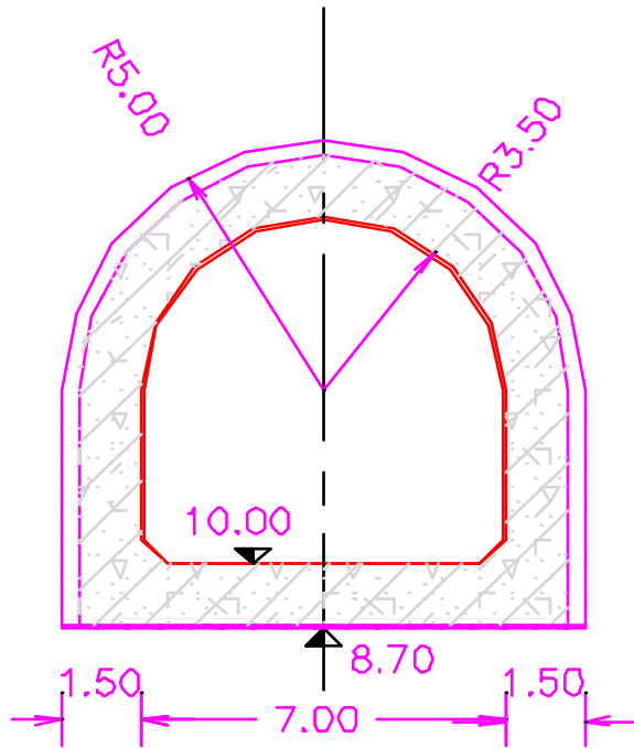
Thân và cửa ra tuynel khi dẫn dòng thí công
