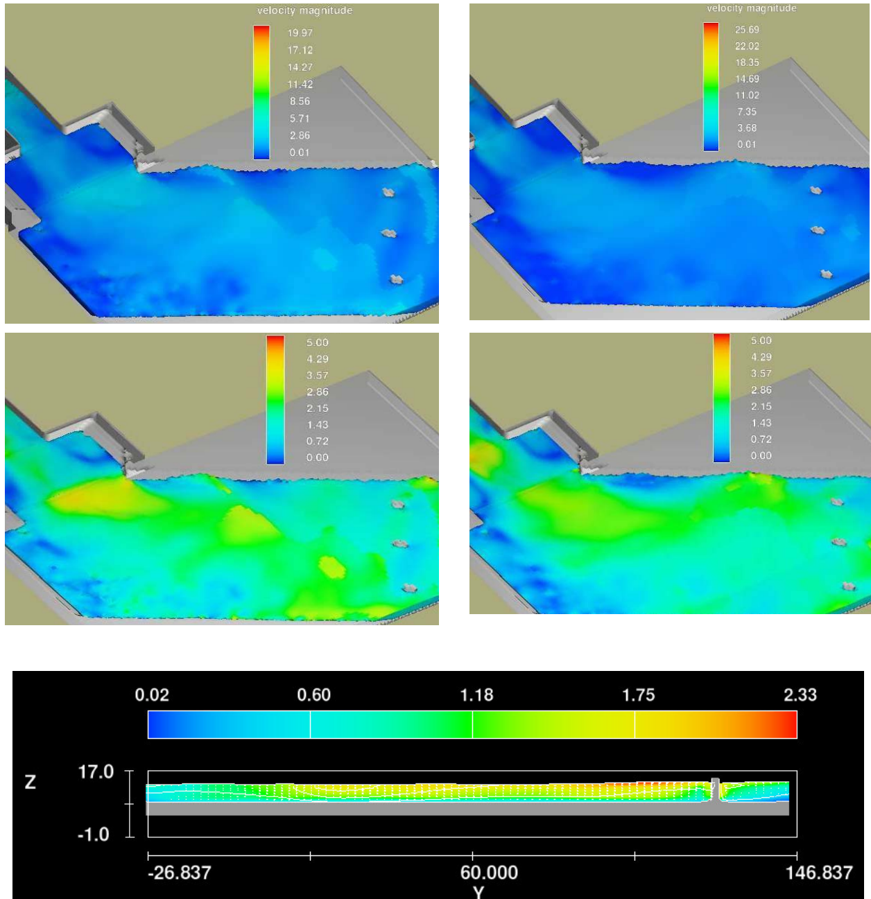
Hình 12. Phân bố và giá trị lưu tốc quá trình dòng chảy qua tuynel ra sông và cầu Ngàn Trươi – trường hợp xả lũ sự cố: , Z_{TL}=Z_{ng\grave{a}n\grave{a}n}=48.2m , Z_{HL}=13.50m ; Q=360m^3/s
