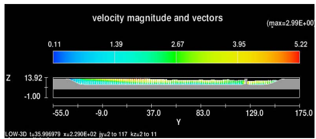
Hình 9. Phân bố và giá trị lưu tốc quá trình dòng chảy qua tuynel ra sông và cầu Ngàn Trươi – trường hợp DDTC 0.5%. Z_b=+0\text{m} ; Z_{TL}=39.5\text{m} ; Z_{HL}=10.93\text{m}
