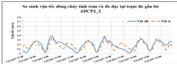
Hình 7: So sánh giữa vận tốc dòng tính toán và đo đạc tại WaveP2_2
