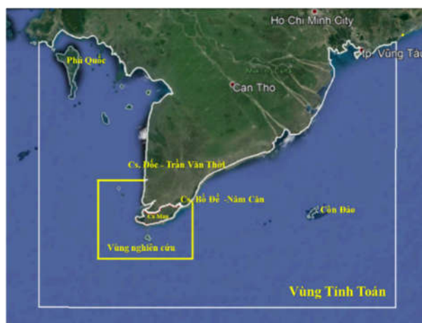
Hình 2: Vùng nghiên cứu chính và vùng tính toán
