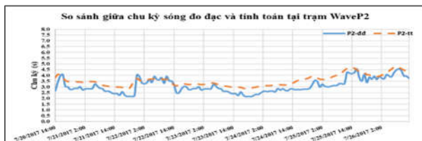
Hình 9: So sánh giữa chu kỳ sóng tính toán và đo đạc tại trạm WaveP2
