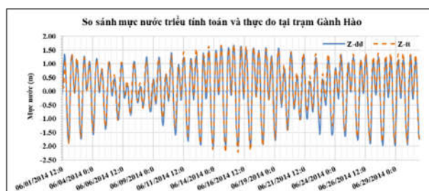
Hình 5: So sánh giữa mực nước tính toán và đo đạc tại trạm Gành Hào
