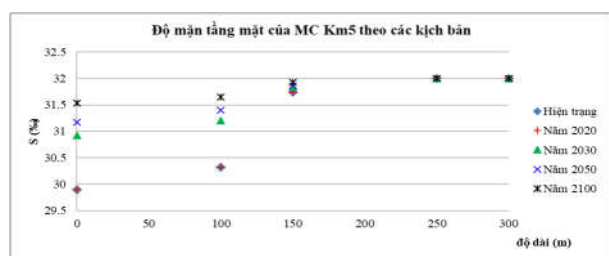
Hình 21: Kết quả độ mặn tăng mặt cắt km5 theo các kịch bản
