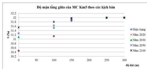
Hình 22: Kết quả độ mặn tăng giữa mặt cắt km5 theo các kịch bản
