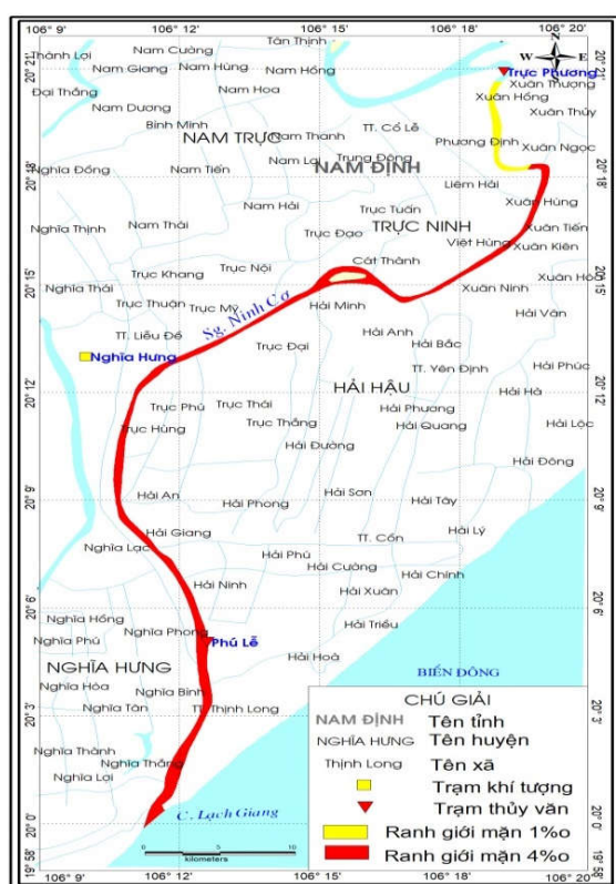
Hình 15: Minh họa kịch bản xâm nhập mặn sông Ninh Cơ kịch bản năm 2030
