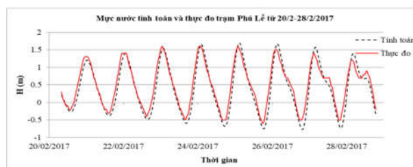
Hình 3: Kết quả hiệu chỉnh mực nước thực đo và tính toán trạm Phú Lễ
