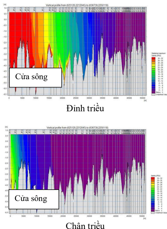
Hình 14: Diễn biến độ mặn lớn nhất, nhỏ nhất dọc sông Ninh Cơ kịch bản hiện trạng
