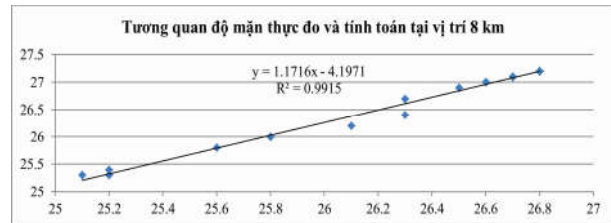
Hình 6: So sánh độ mặn thực đo và tính toán tại mặt cắt vị trí 8 km
