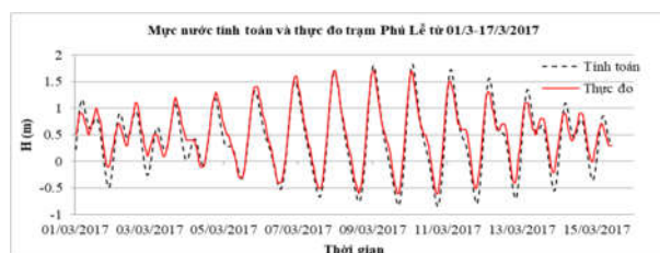
Hình 4: Kết quả kiểm định mực nước thực đo và tính toán trạm Phú Lễ
