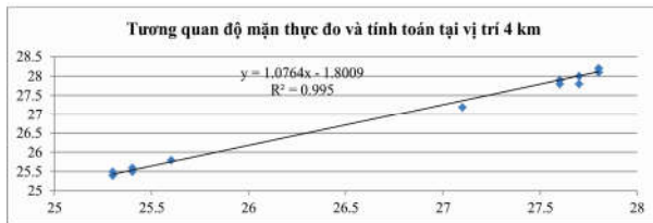
Hình 5: So sánh độ mặn thực đo và tính toán tại mặt cắt vị trí 4 km
