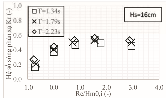
Hình 3.12: Ảnh hưởng của R_c/H_{m0,i} tới K_t , K_r ứng với các chu kỳ sóng khác nhau
