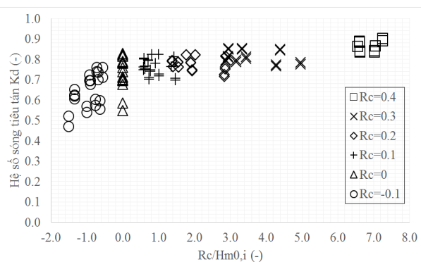
Hình 3.9: Tương quan giữa K_d và R_c/H_{m0,i} ứng với các giá trị chiều cao lưu không
