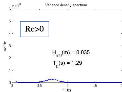
(d) Phổ sóng sau công trình
