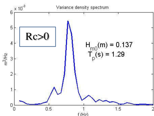
(c) Phổ sóng trước công trình
