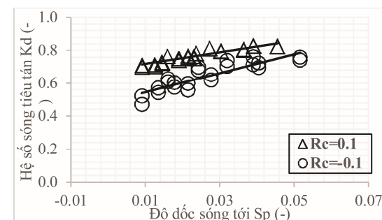
(f) Quan hệ K_d-S_p
