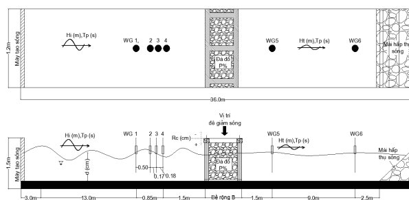
Hình 2.4: Bố trí kim đo sóng trong máng sóng
