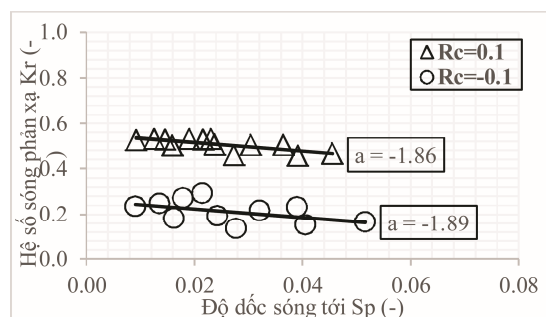
(d) Quan hệ K_r-S_p
