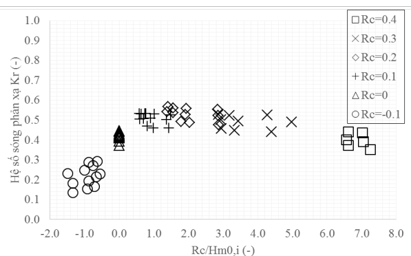
Hình 3.8: Tương quan giữa K_r và R_c/H_{m0,i} ứng với các giá trị chiều cao lưu không
