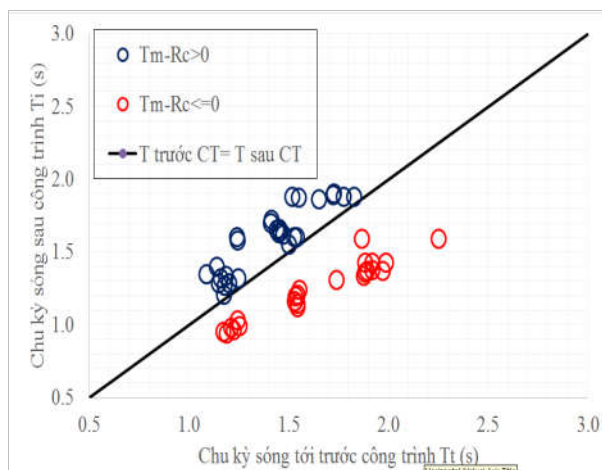
Hình 3.5: Biến đổi chu kỳ phổ trung bình T_m trước và sau công trình
