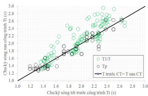
Hình 3.4: Biến đổi chu kỳ đỉnh phổ T_p ; T_{1/3} trước và sau công trình
