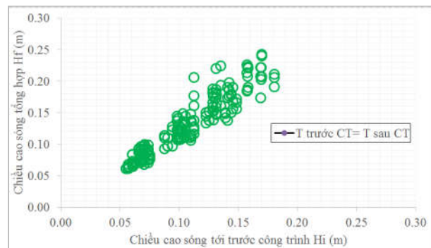
Hình 3.6: Biến đổi sóng tổng hợp trước công trình so với sóng tới
