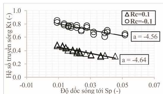
(b) Quan hệ K_r-S_p
