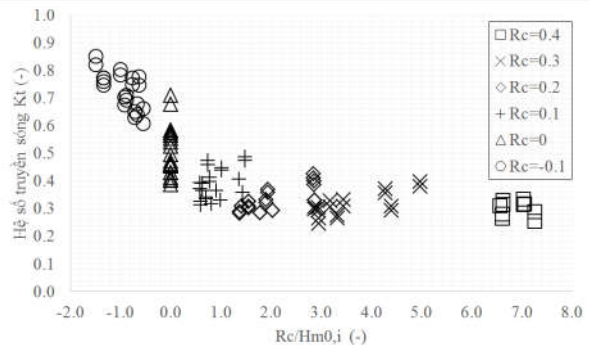
Hình 3.7: Ảnh hưởng của R_c/H_{m0,i} đến K_t ứng với các giá trị chiều cao lưu không
