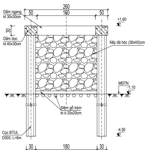
Hình 2.2: Kích thước công trình thực tế
