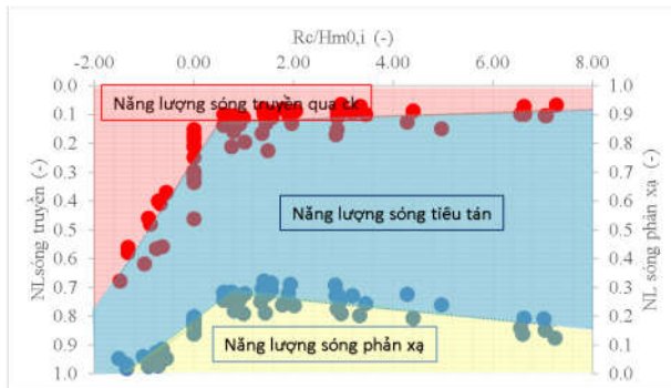
Hình 3.10: Sự biến đổi năng lượng sóng khi tương tác với kết cấu ứng với giá trị chiều cao lưu không định đề tương đối R_c/H_{m0,i}
