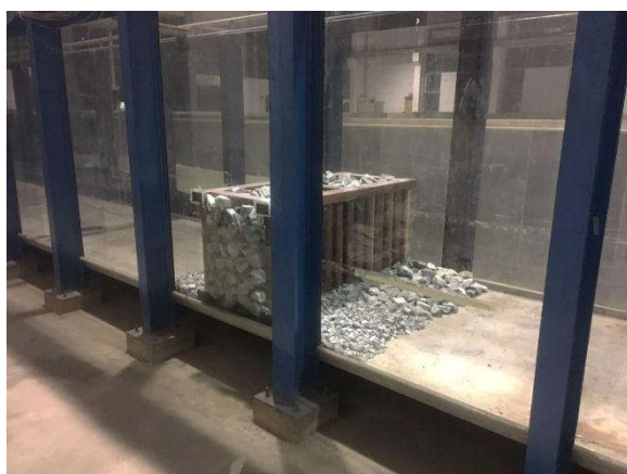
Hình 2.3: Mô hình thí nghiệm theo tỷ lệ 1/5
