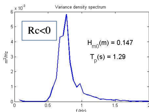
Hình 3.3: Sự biến đổi phổ năng lượng sóng khi truyền qua cấu kiện
