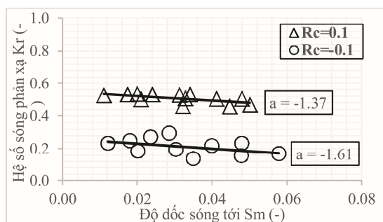
(c) Quan hệ K_r-S_m
